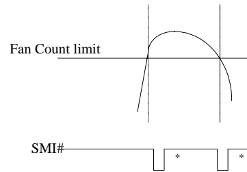
Figure 15-2. Fan SMI# Mode
